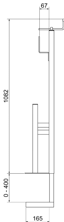
Abb. / Fig. 6: Maße / dimensions 111932 / 111932V
