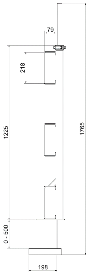
Abb. / Fig. 7: Maße / dimensions 111933
