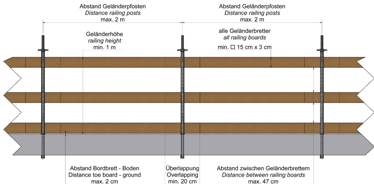
Abb. / Fig. 2: maßliche Vorschriften / dimensional regulations
