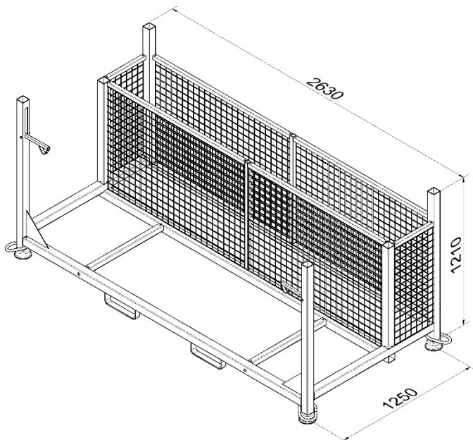
Abb. / Fig. 11: Maße / Dimensions 112960-5
